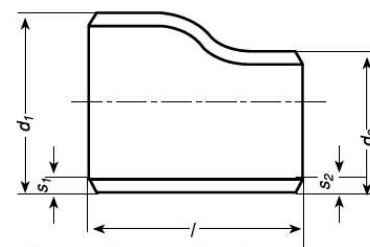
Eccentric reducer / Ексцентричен преход
