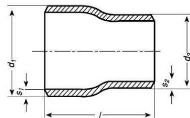
Concetric reducer / Концентричен преход
